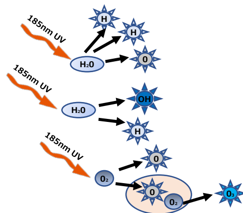
UV-C 185nm商社によるフリーラジカル生成イメージ
