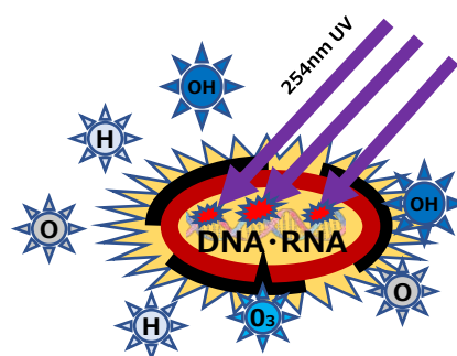
UV-C 254nm照射によるDNA・RNA直接損傷イメージ
